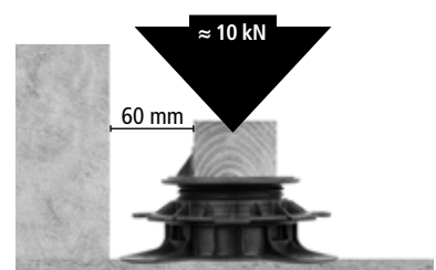
Wandanschluss + Tragkraft
