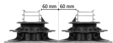
Stoßausführung
